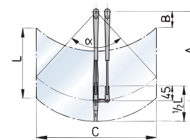
Wischerblatt am oberen Befestigungspunkt des Armes.
