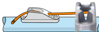
CL702 / CL702AN mit gewölbter Basis CL702 / CL702AN with curved base
